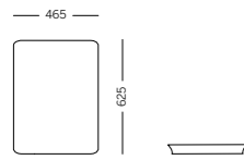
MODULO T1 - Tavolo piccolo rettangolare MODULE T1 - Small rectangular table
