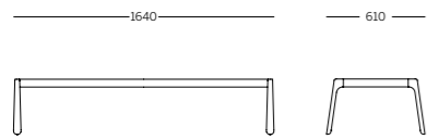
MODULO C - Struttura per 3 unità MODULE C - Structure for 3 units
