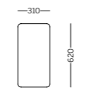
MODULO T2 - Top tavolino rettangolare, ½ unità MODULE T2 - Rectangular table top, ½ unit
