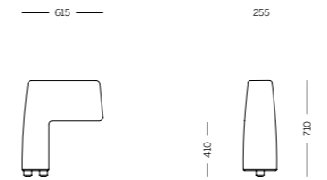
MODULO M - Bracciolo MODULE M - Armrest
